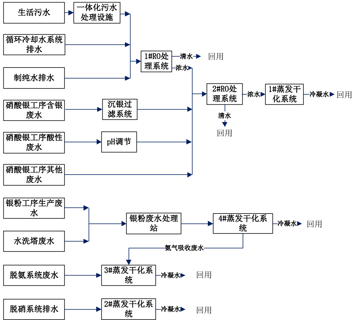
图 3-1 项目废水处理措施和去向示意图
