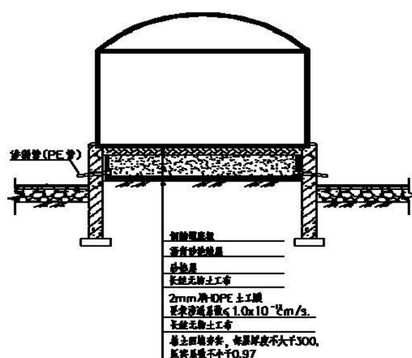
图 7-16 环墙式罐基础防渗
