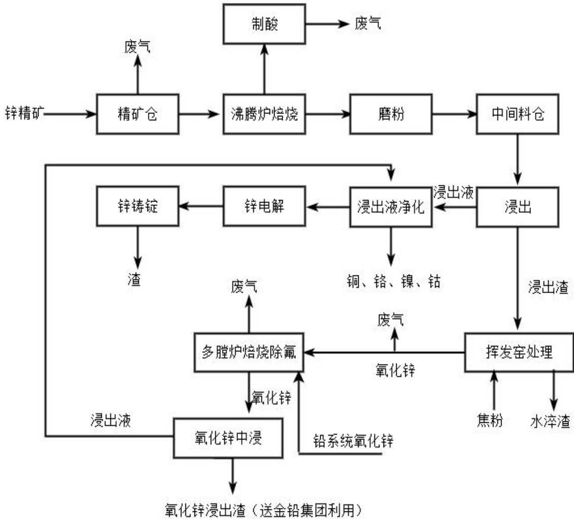
图 4-1 生产工艺流程图
